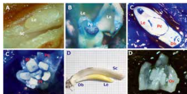
図1 図. カタクリ球根内部構造。A, 5/10; B, 7/26; C, 9/13; D, 11/14 Sc: 鱗片葉原基, Le: 葉原基, Pe: 花被, St: 雄蕊, P: 雌蕊, Ov: 胚珠, Db: 主球根
