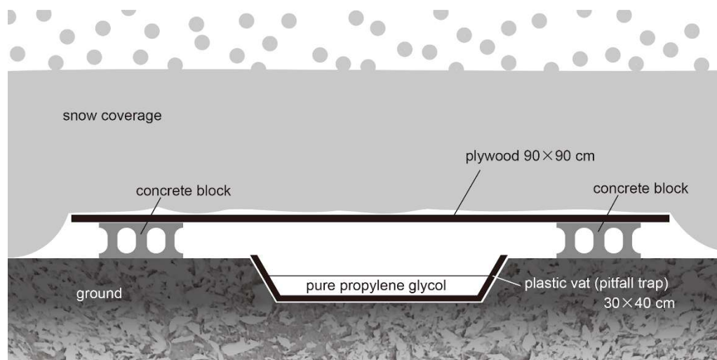
図1. 落とし穴トラップの断面図。雪と地面の間を歩き回る虫が、地面と同じ高さになるように埋めたプラスチック製バットの中に落ちる仕組みです。バットの周辺にコンクリートブロックを置き、その上にベニヤ板をかぶせることで、バットが雪に埋もれることを防いでいます。バットの中には非誘因性の不凍液（プロピレングリコール）が入っており、バットの中に落ちた虫が保存されます。
